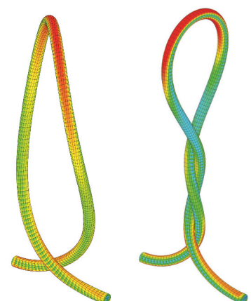
Instabilité d'une corde sous flambage élastique en torsion
