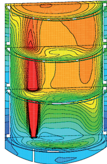
Outil Métier pour l'analyse du risque H 2 dans une enceinte
